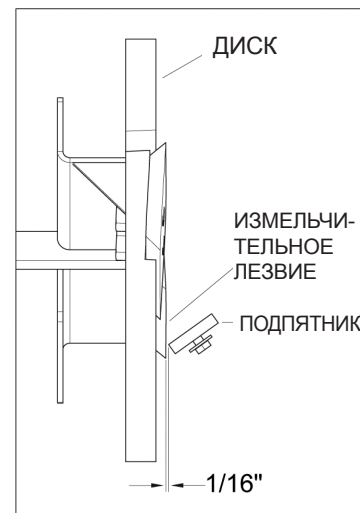
Рис. 5.2. Зазор между измельчительным лезвием и измельчительным подпятником
