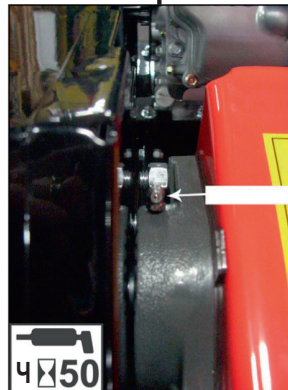
Передней подшипник ротора
