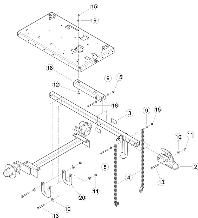
Рис. 2.7. Узел в разобранном виде для демонстрации конструкции
