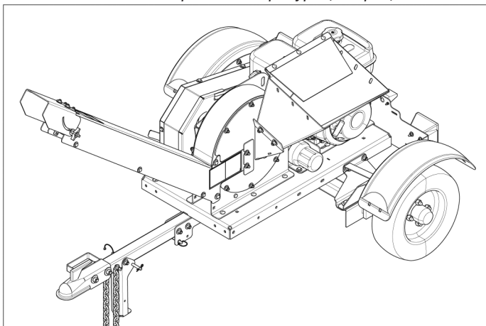
Рис. 2.10. Вариант конфигурации прицепа
