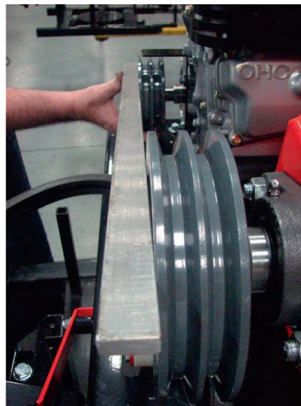
Рис. 5.7. Проверка центровки шкива
