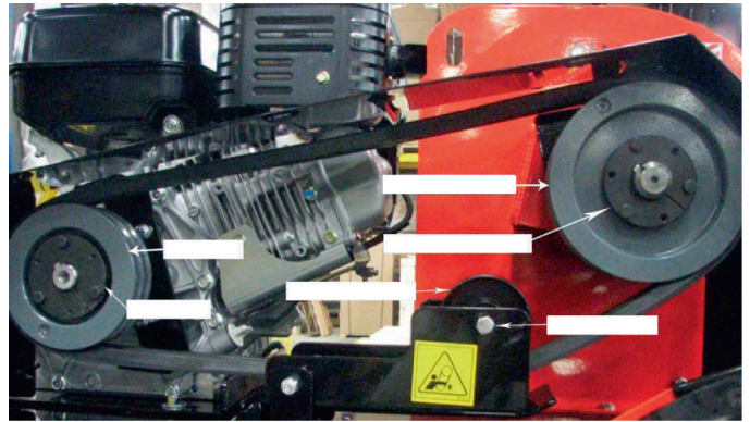
Рис. 5.6. Замена приводного ремня
